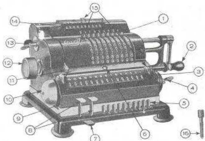
Fig. 33. Facit-räknemaskin.
